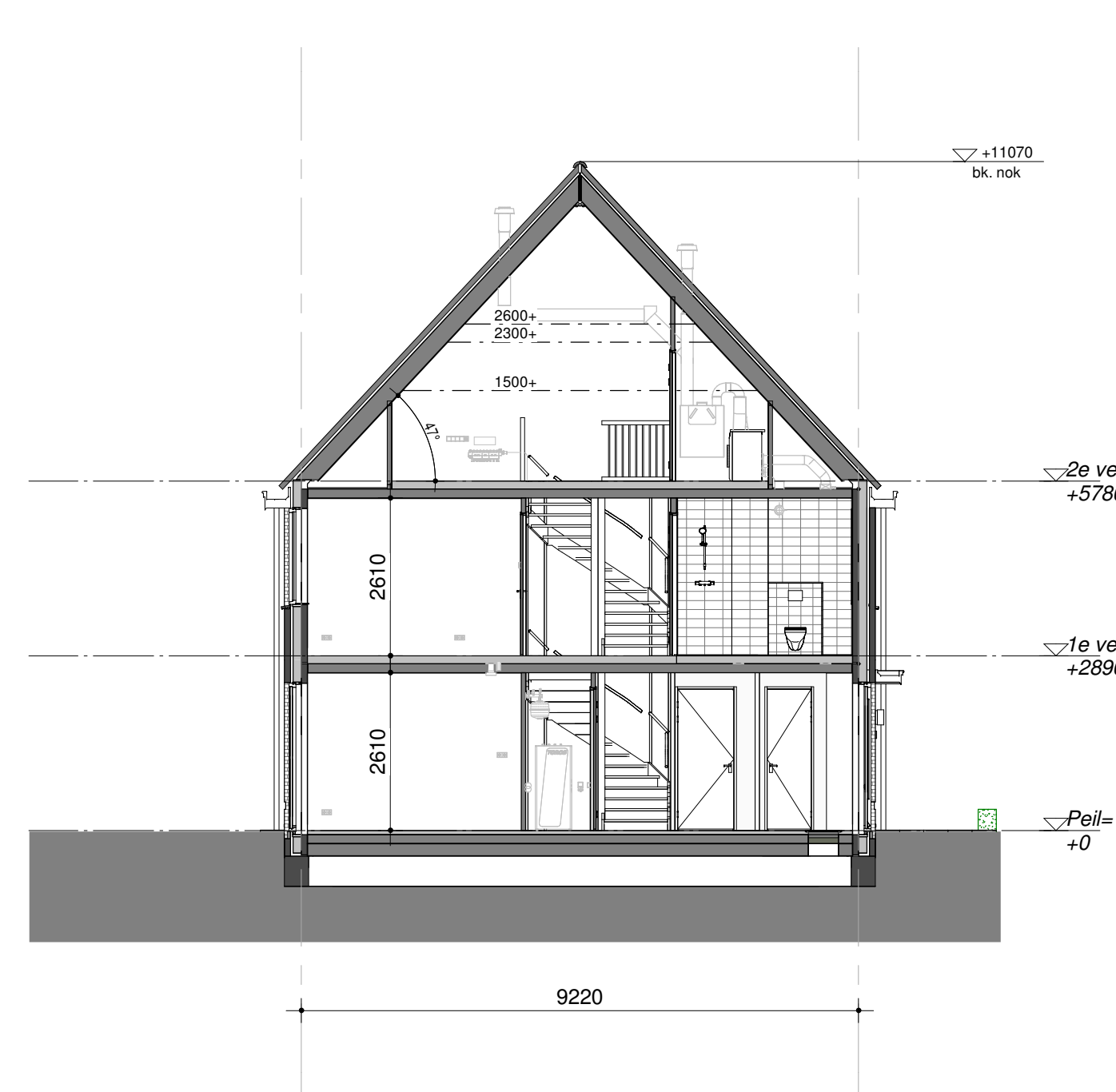
Doorsnede Schaal: 1 : 100
